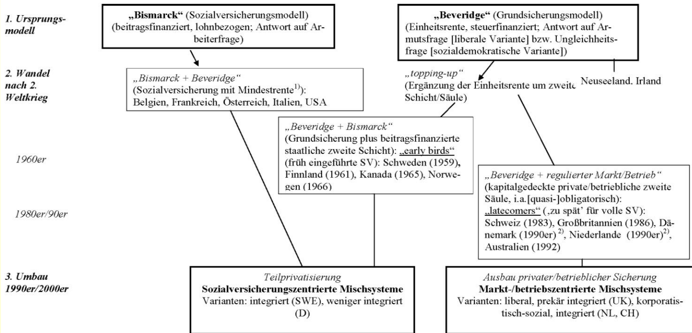
Schaubild 1: Strukturwandel der Alterssicherungsarrangements in westlichen Ländern
